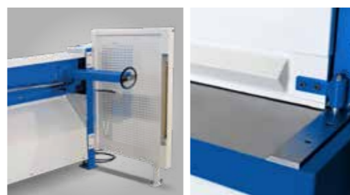
Rückraum durch Lichtschranke abgesichert
